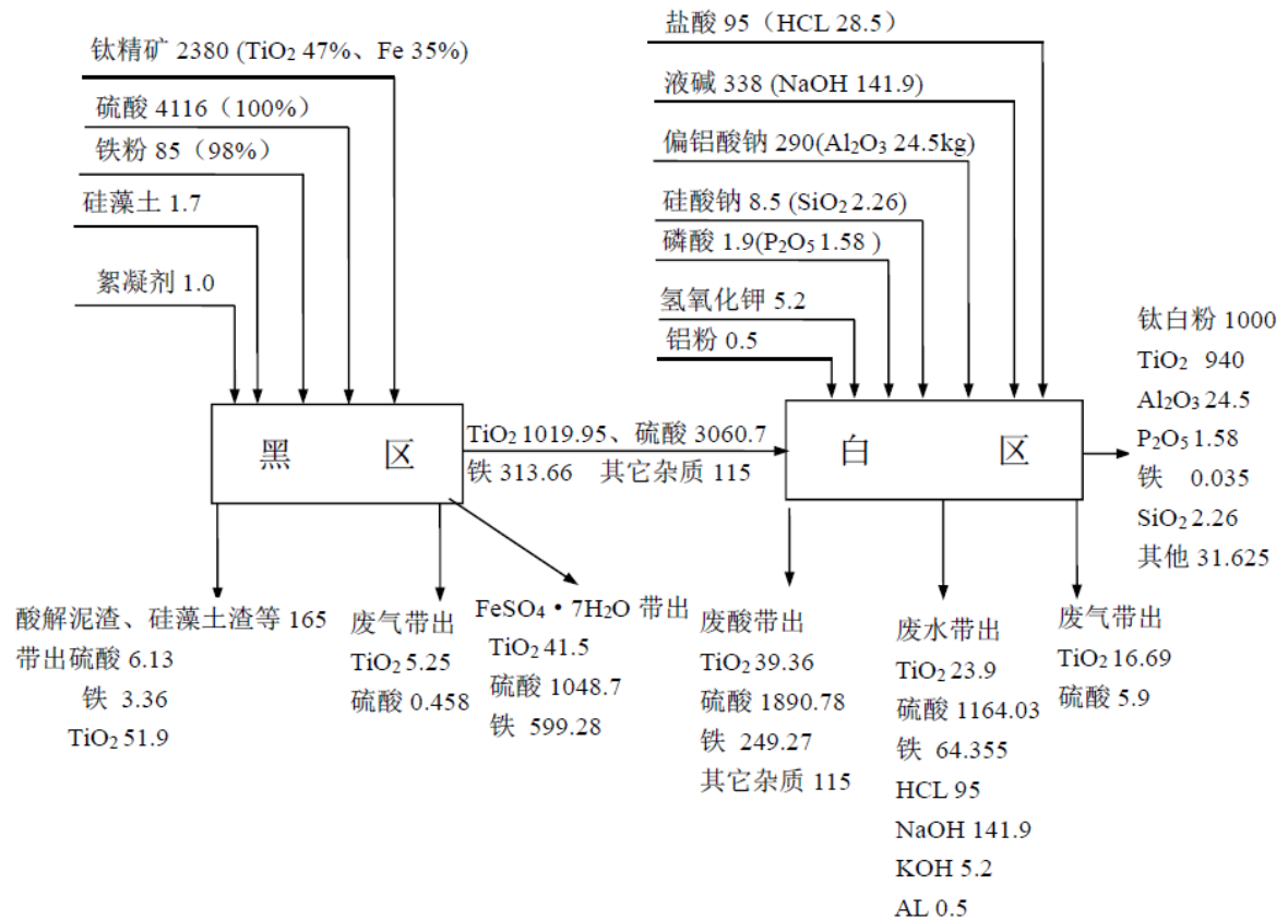
图 2.1-9 钛白粉生产装置总物料平衡图 （单位：kg/t 钛白粉）
