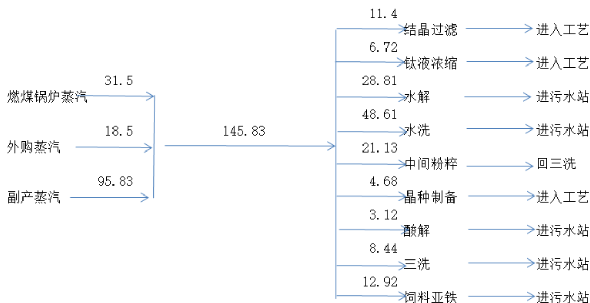
图 2.3-4 蒸汽平衡图 单位: t/h
