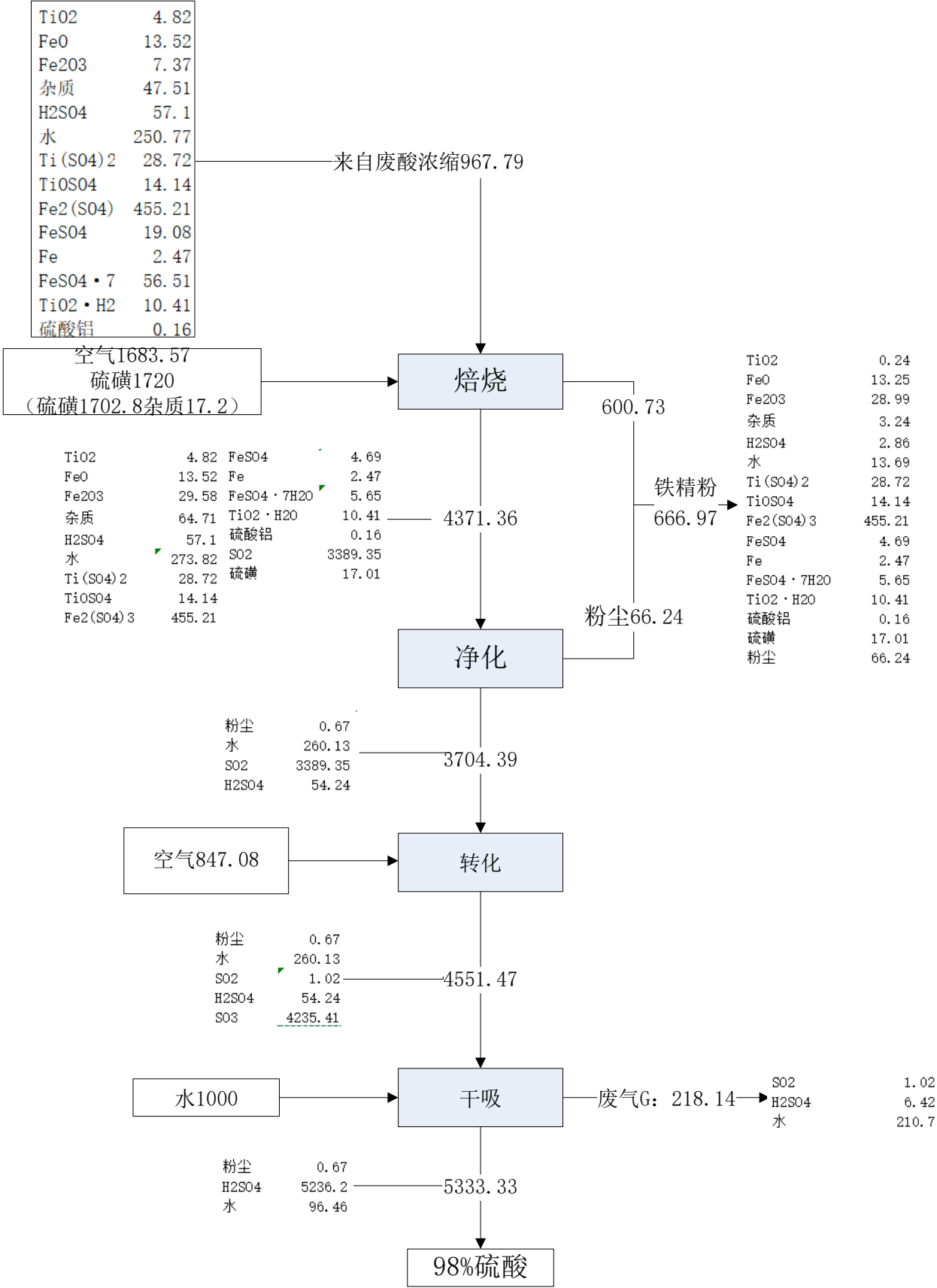
图 2.3-4 硫酸装置物料平衡及元素平衡图 单位: kg/t 钛白粉
