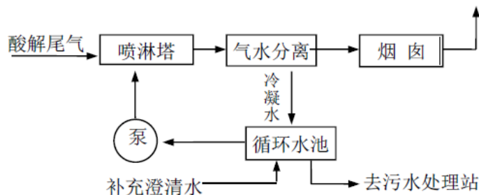
图 6.1-1 酸解尾气处理流程图
