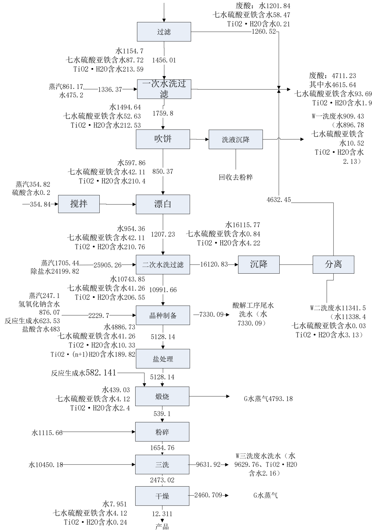
图 2.3-2 钛白粉装置水平衡图 单位: kg/t 钛白粉
