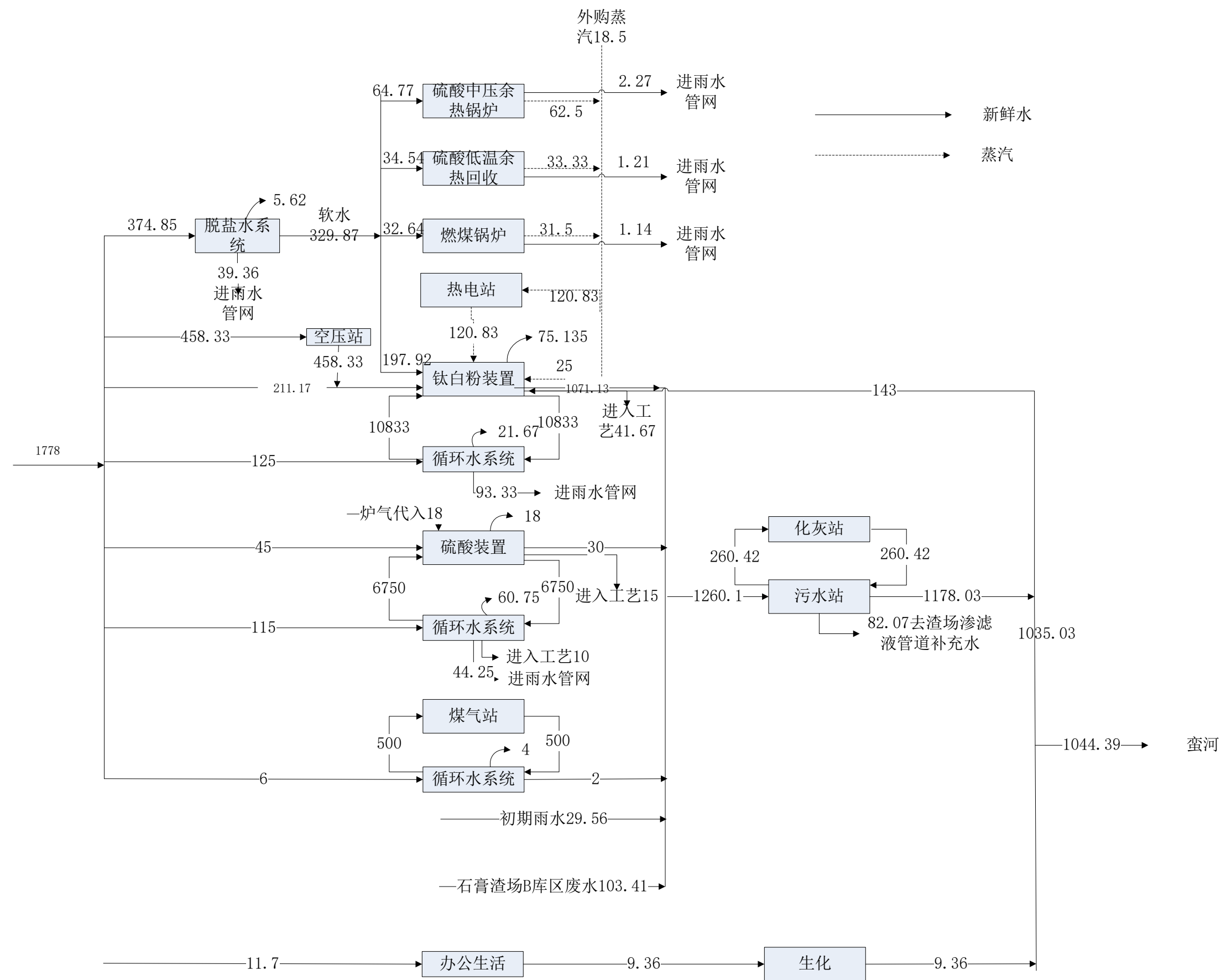
图 2.3-4 项目水平衡图 单位: m³/h
