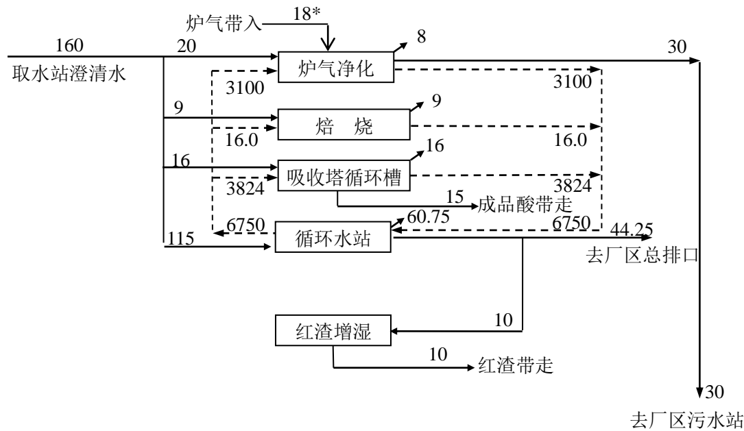
图 2.3-3 硫酸装置水平衡图(单位: m 3 /h)
