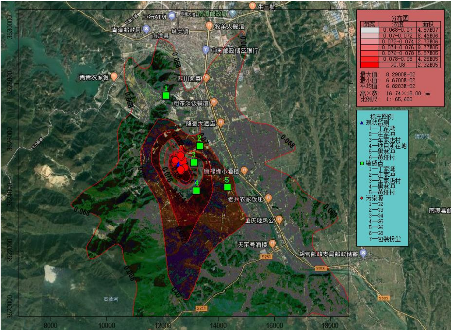
图 5.1-4b 未叠加背景值后 PM2.5 二次污染物最大落地浓度日平均浓度贡献值等浓度线图
