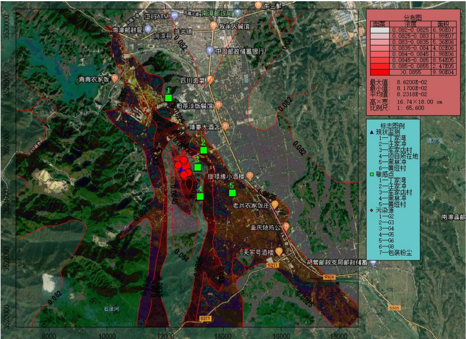
图 5.1-8a 叠加背景值后 PM 10 最大落地浓度日平均浓度贡献值等浓度线图
