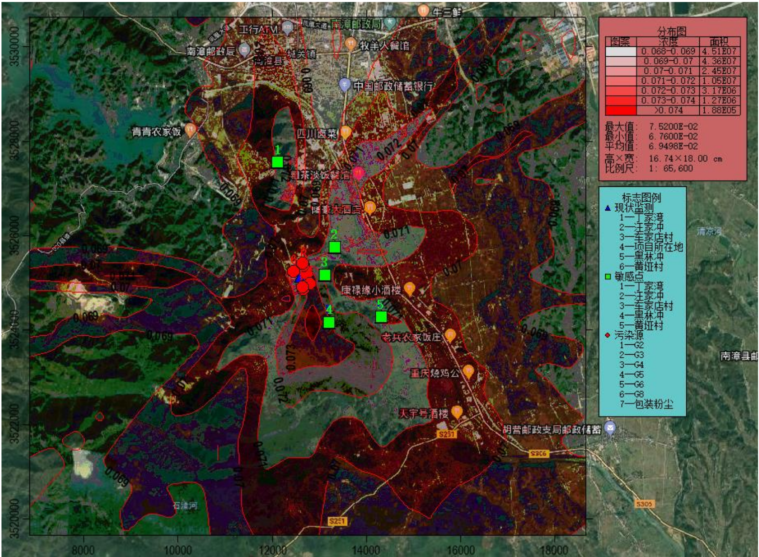
图 5.1-1a 叠加背景值后 PM2.5 一次污染物最大落地浓度小时平均浓度贡献值等浓度线图
