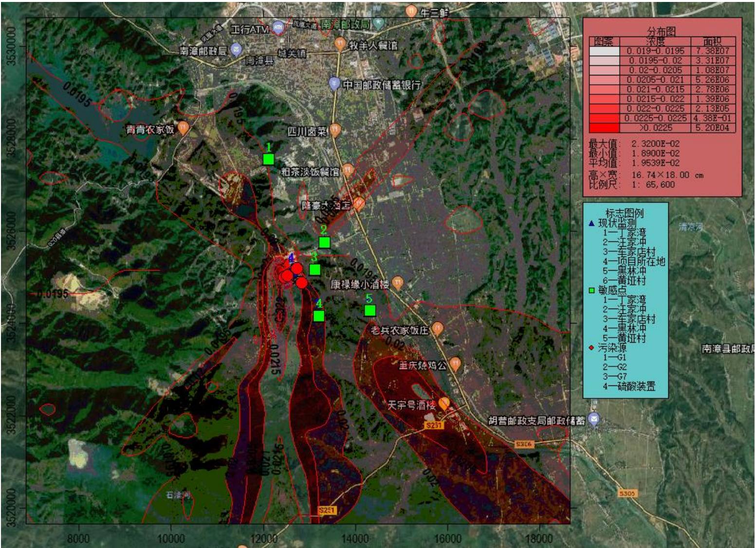
图 5.1-10b 叠加背景值硫酸雾最大落地浓度日平均浓度贡献值等浓度线图
