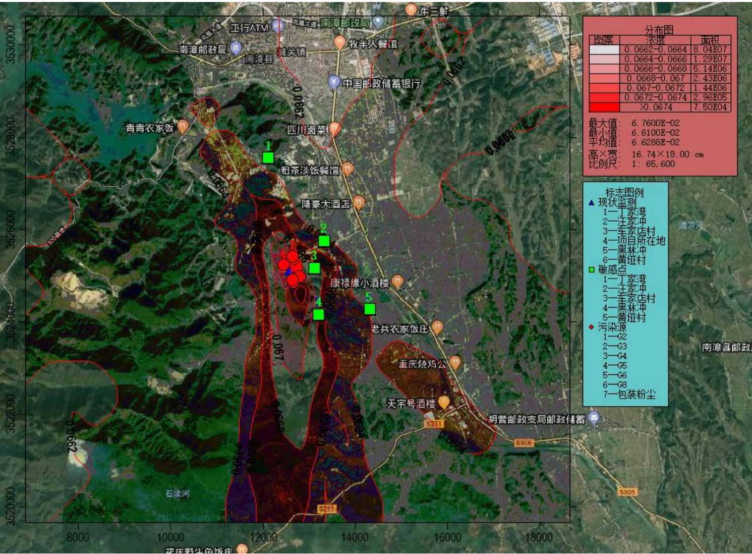
图 5.1-1b 叠加背景值后 PM2.5 一次污染物最大落地浓度日平均浓度贡献值等浓度线图
