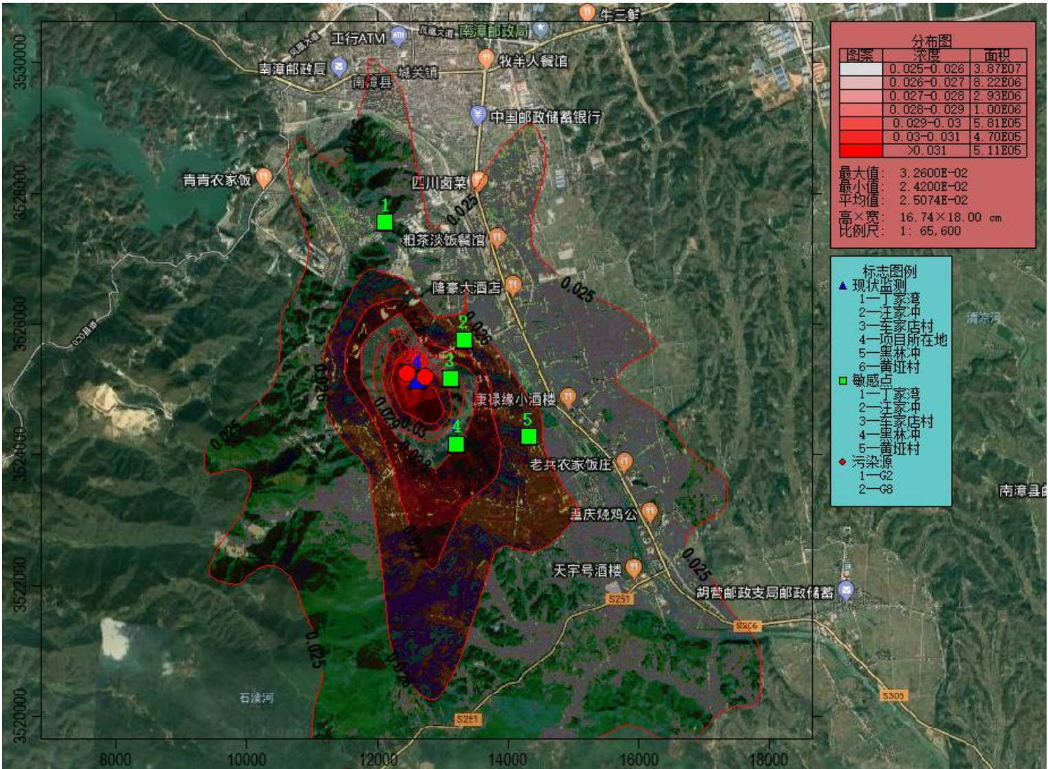
图 5.1-7b 叠加背景值后 NO 2 最大落地浓度日平均浓度贡献值等浓度线图
