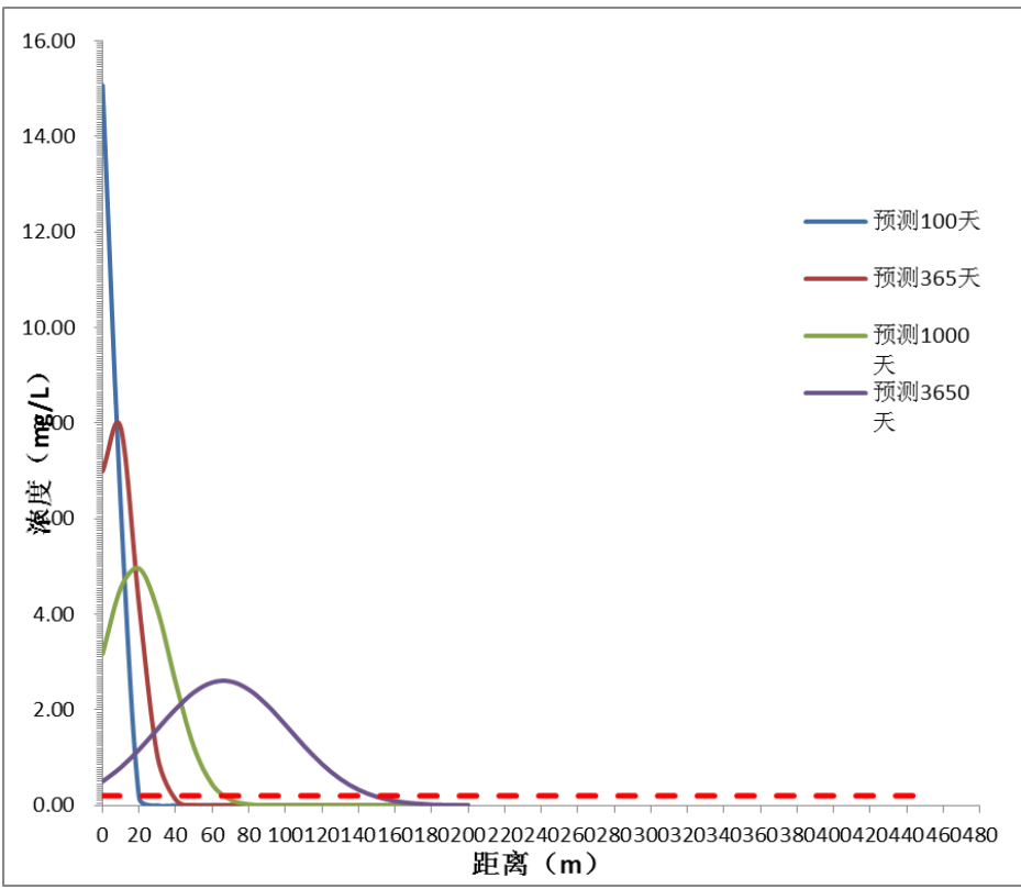
图 5.4-8 磷酸盐迁移图
