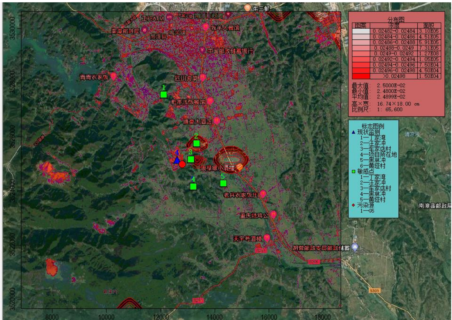
图 5.1-5a 叠加背景值后 HCl 最大落地浓度小时平均浓度贡献值等浓度线图
