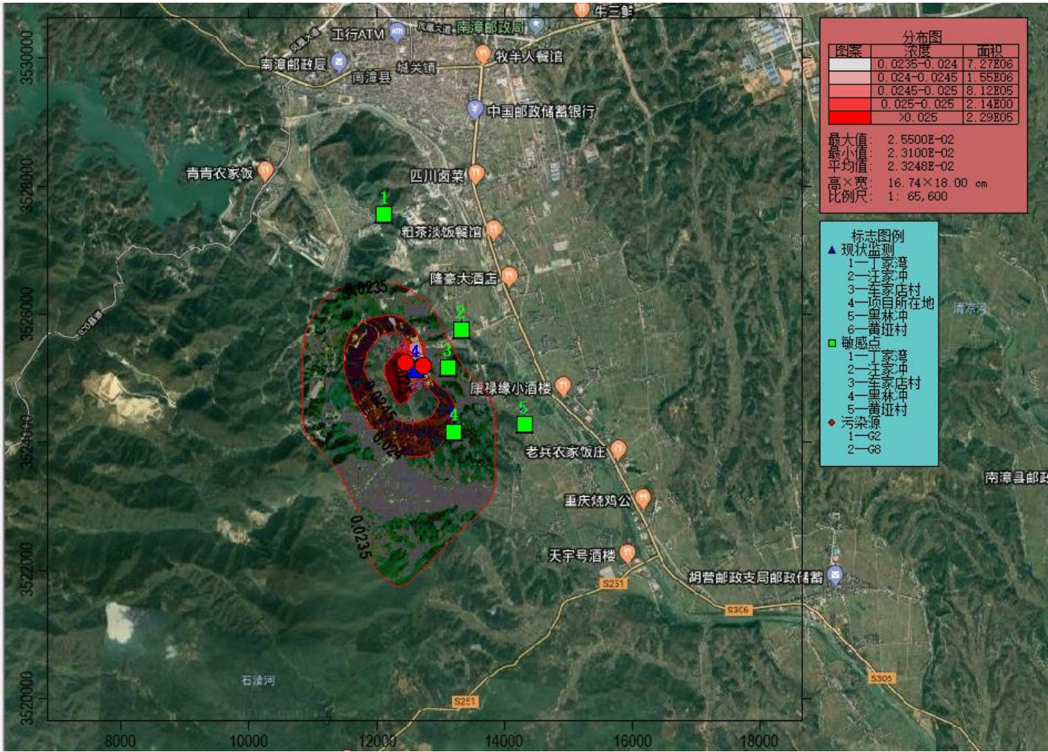
图 5.1-7c 叠加背景值后 NO 2 最大落地浓度年平均浓度贡献值等浓度线图
