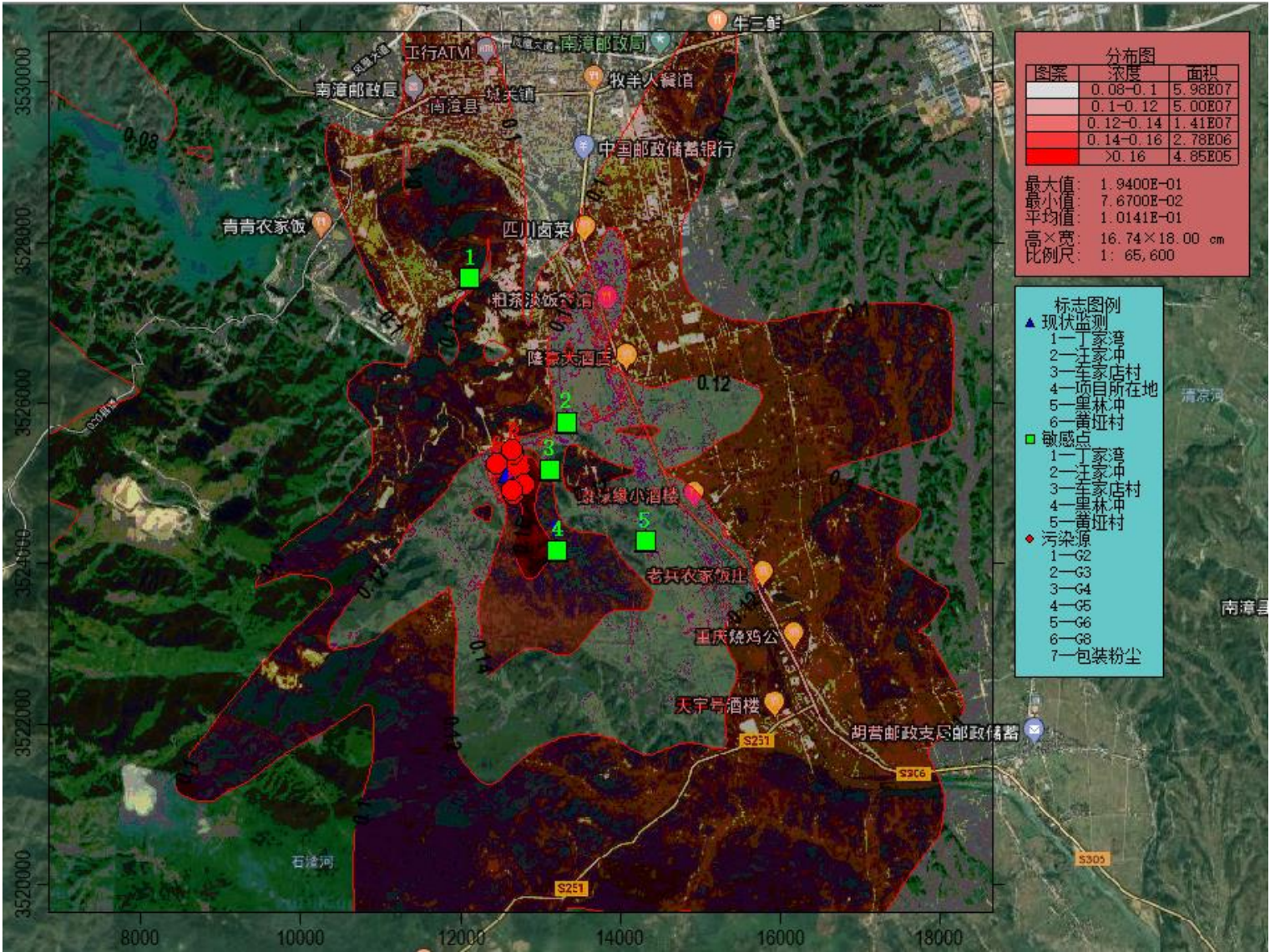
图 5.1-3c 叠加背景值后 PM2.5 二次污染物最大落地浓度年平均浓度贡献值等浓度线图
