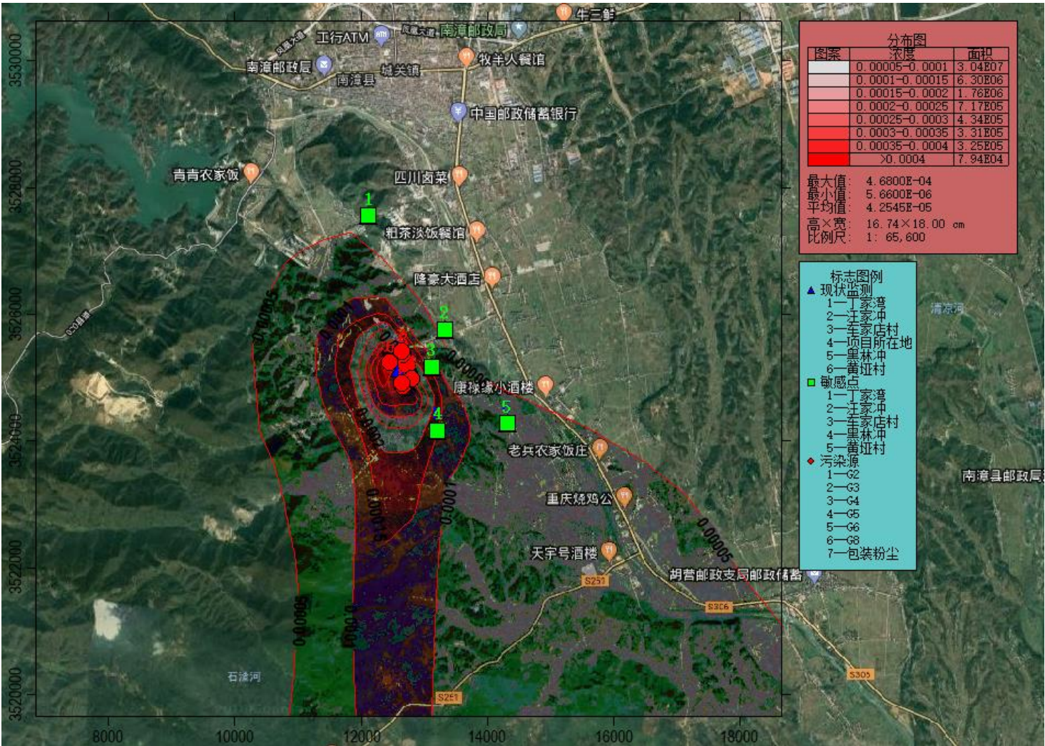
图 5.1-2c 未叠加背景值后 PM2.5 一次污染物最大落地浓度年平均浓度贡献值等浓度线图
