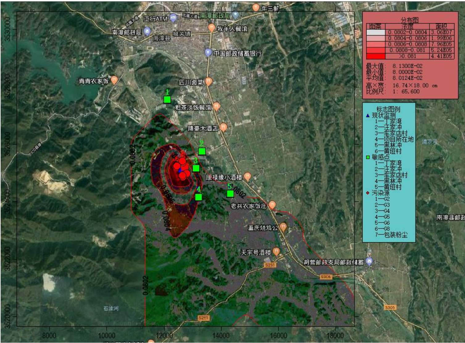
图 5.1-8b 叠加背景值后 PM 10 最大落地浓度年平均浓度贡献值等浓度线图
