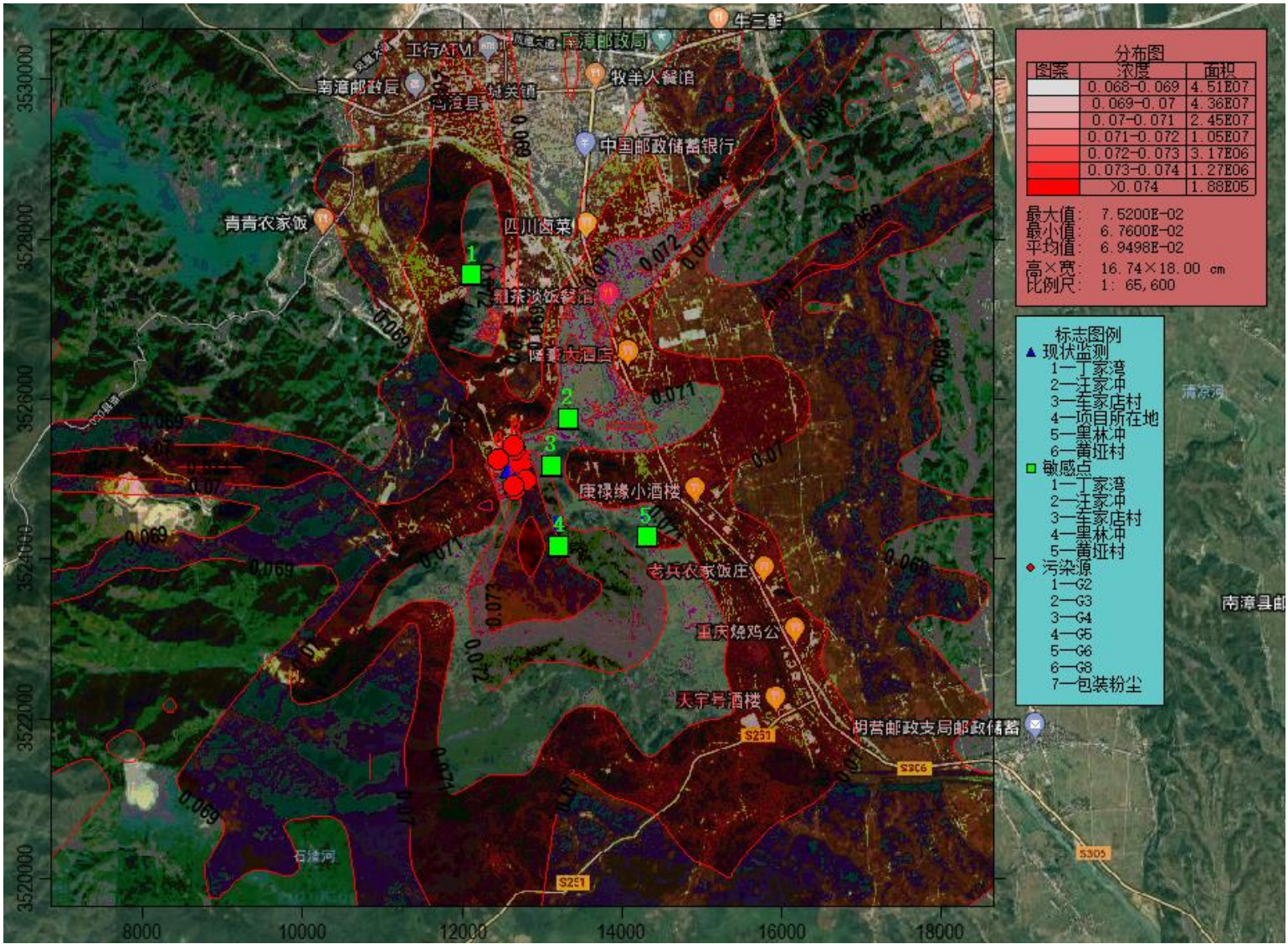
图 5.1-1c 叠加背景值后 PM2.5 一次污染物最大落地浓度年平均浓度贡献值等浓度线图
