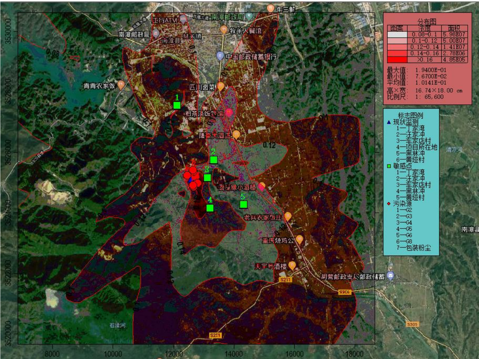
图 5.1-4a 未叠加背景值后 PM2.5 二次污染物最大落地浓度小时平均浓度贡献值等浓度线图
