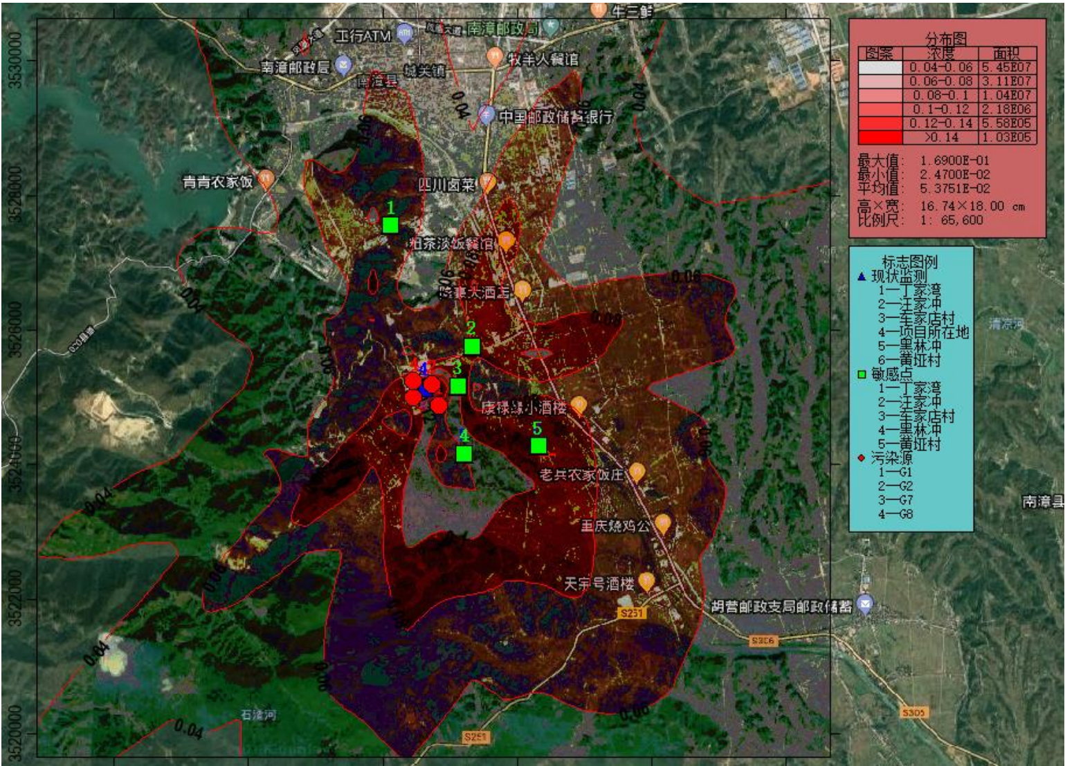
图 5.1-9a 叠加背景值 SO 2 最大落地浓度小时平均浓度贡献值等浓度线图
