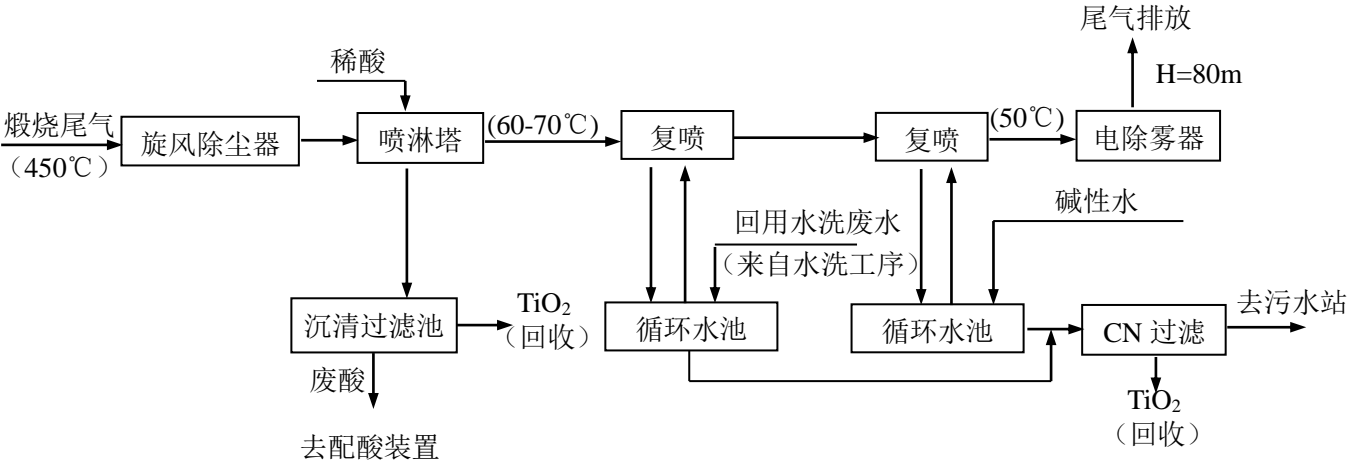
图 6.1-2 煅烧尾气处理流程图
