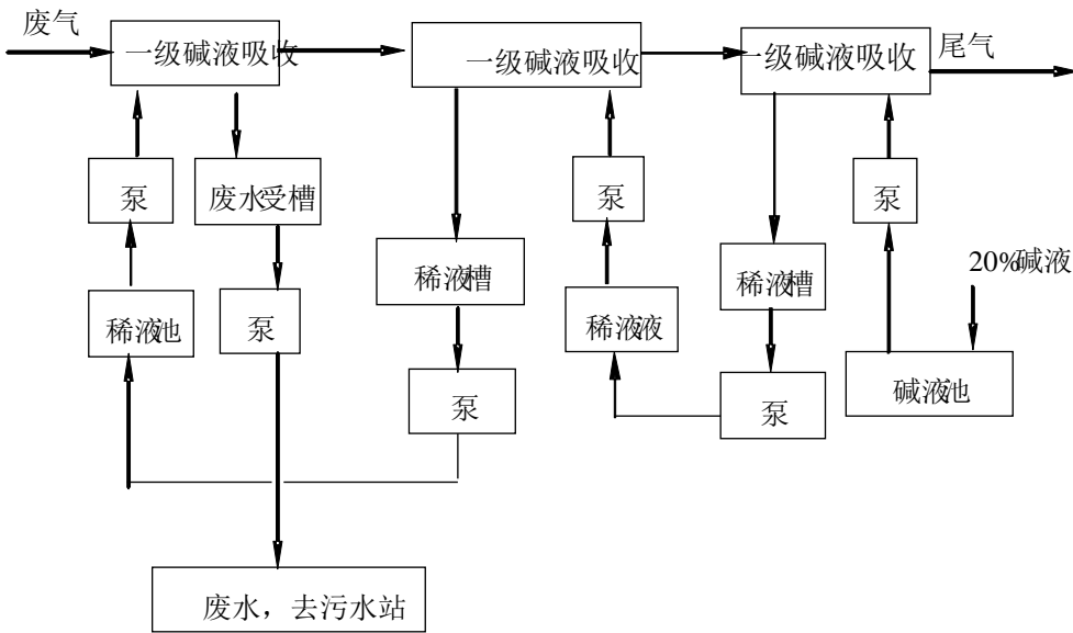
图 6.2-2 三级碱吸收装置流程图
