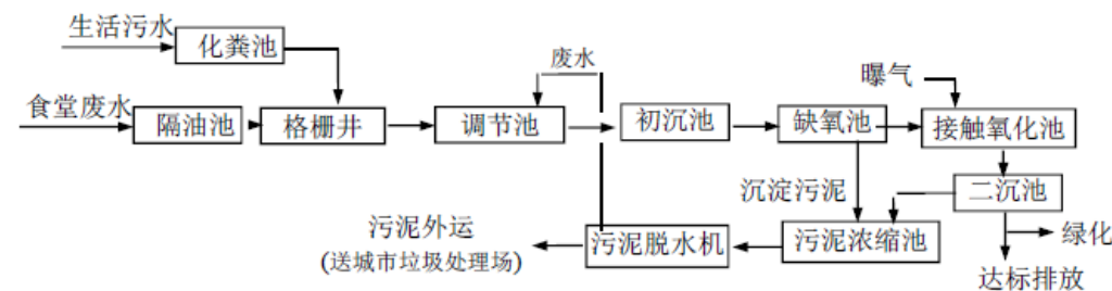
图 6.1-1 生活污水处理工艺流程图
