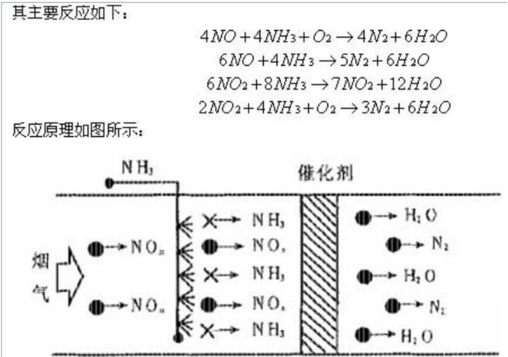
图 6.2-1 SCR 反应原理示意图
