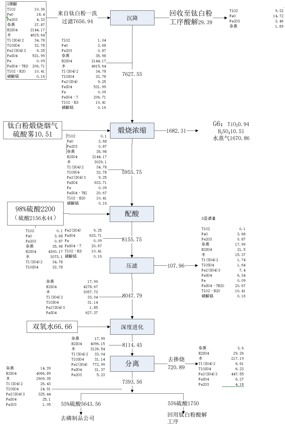
图 2.3-3 废酸浓缩装置物料平衡及元素平衡图 单位: kg/t 钛白粉
