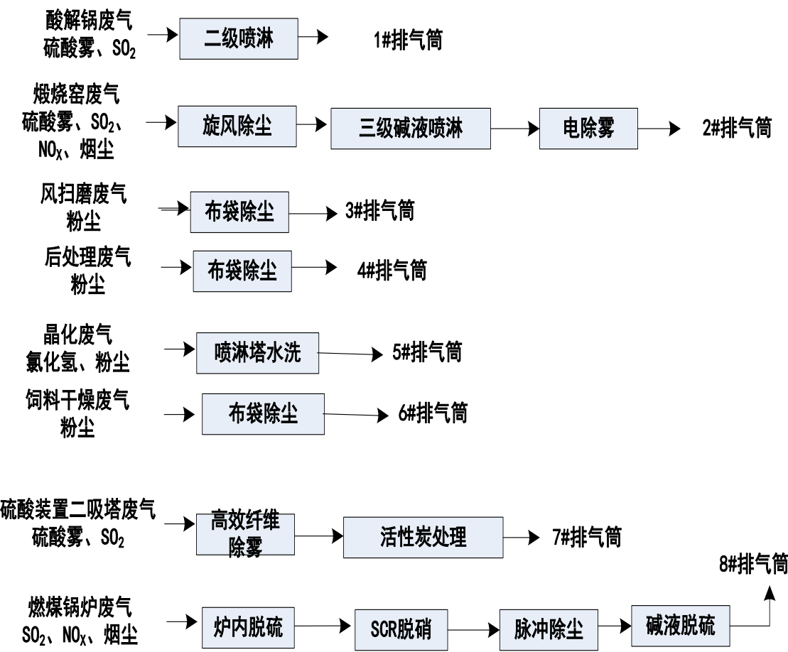
图 6.3-1 废气处理示意图
