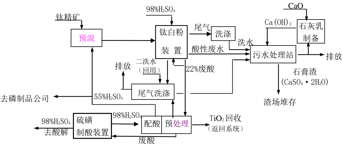
图 8-1 金红石型钛白粉装置污染治理嫁接技术示意图
