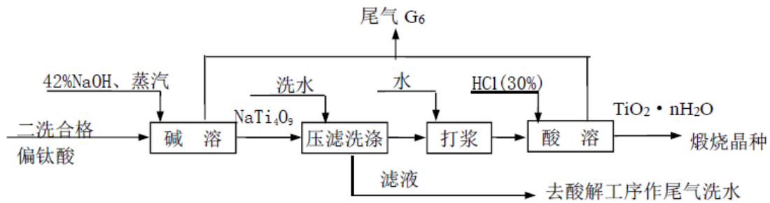
图 2.1-6 煅烧晶种制备工艺
