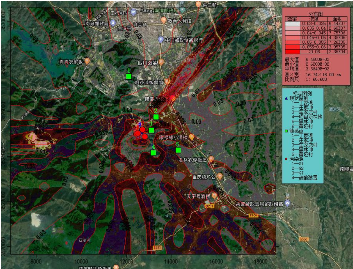
图 5.1-10a 叠加背景值硫酸雾最大落地浓度小时平均浓度贡献值等浓度线图
