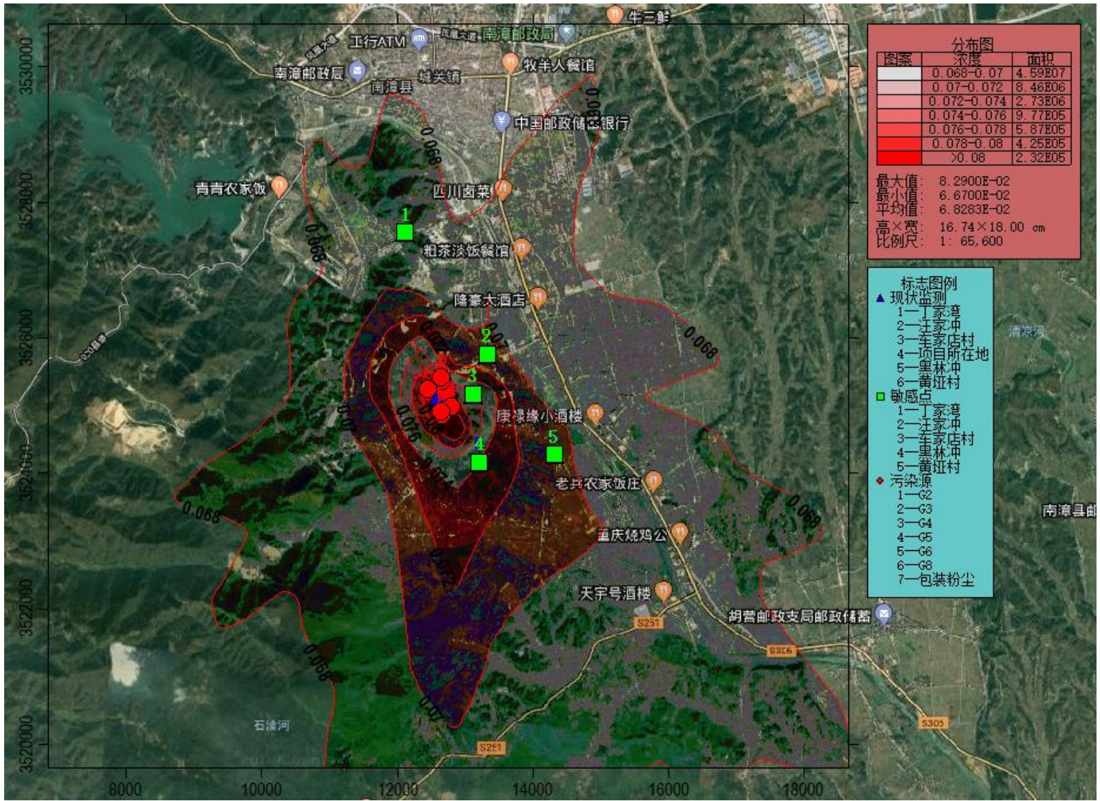
图 5.1-3b 叠加背景值后 PM2.5 二次污染物最大落地浓度日平均浓度贡献值等浓度线图
