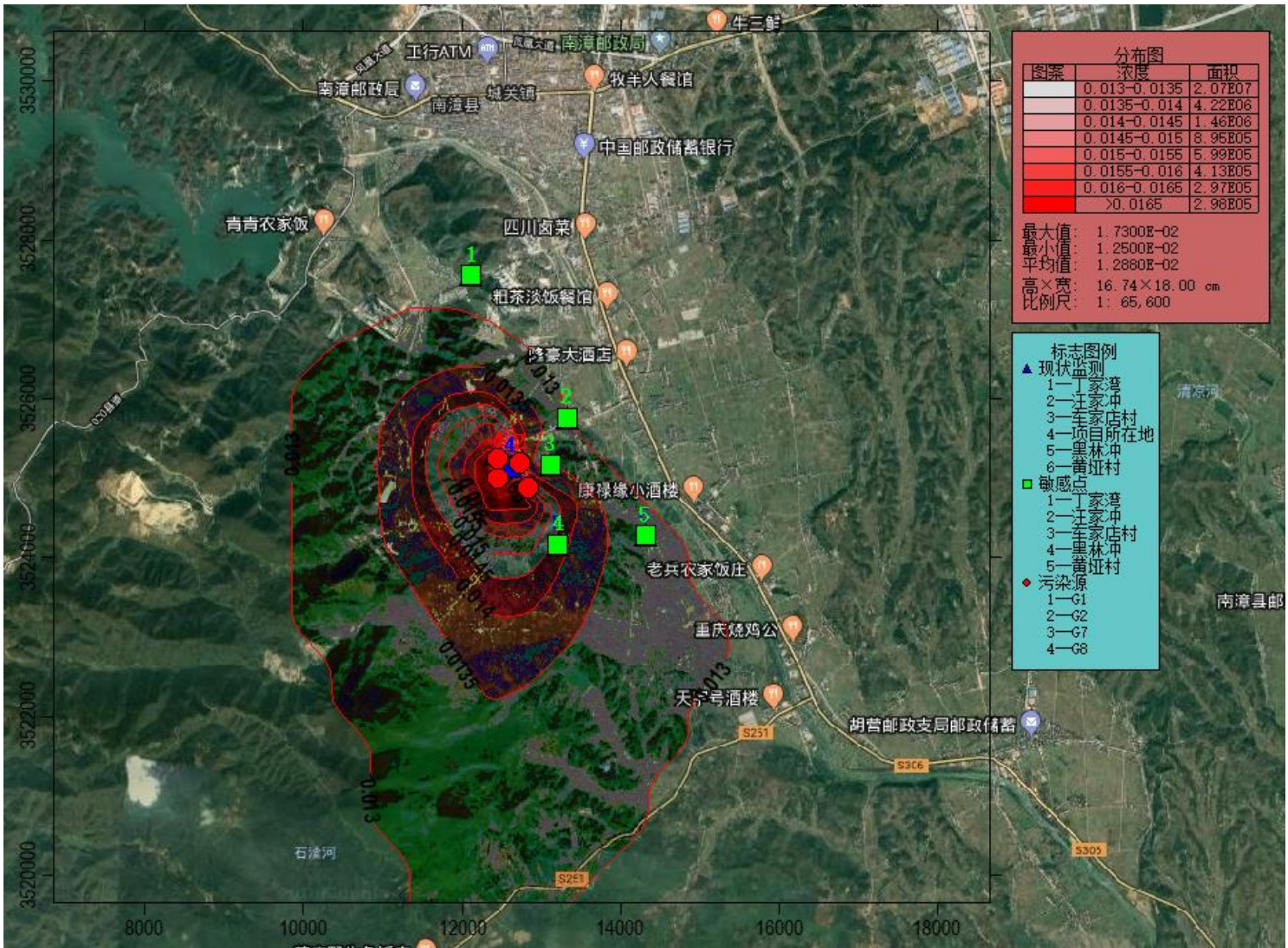
图 5.1-9c 叠加背景值 SO 2 最大落地浓度年平均浓度贡献值等浓度线图
