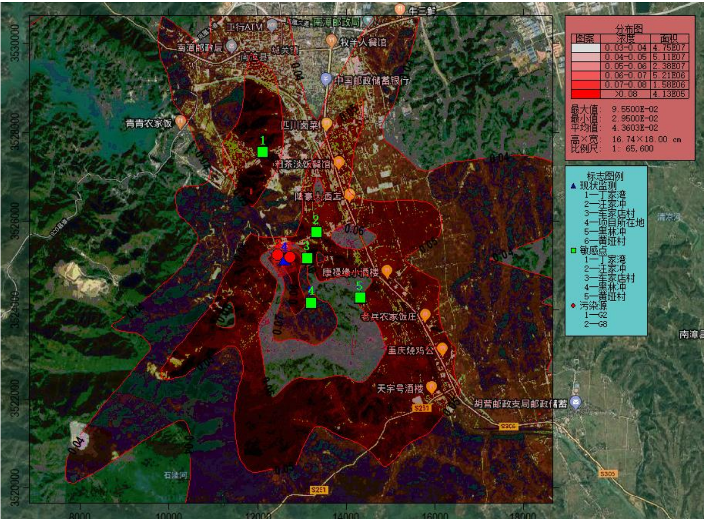
图 5.1-11c 非正常工况叠加背景值 NO 2 最大落地浓度小时平均浓度贡献值等浓度线图
