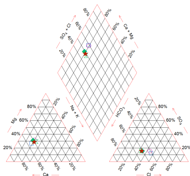
5.4-4 地下水水化学三线图
