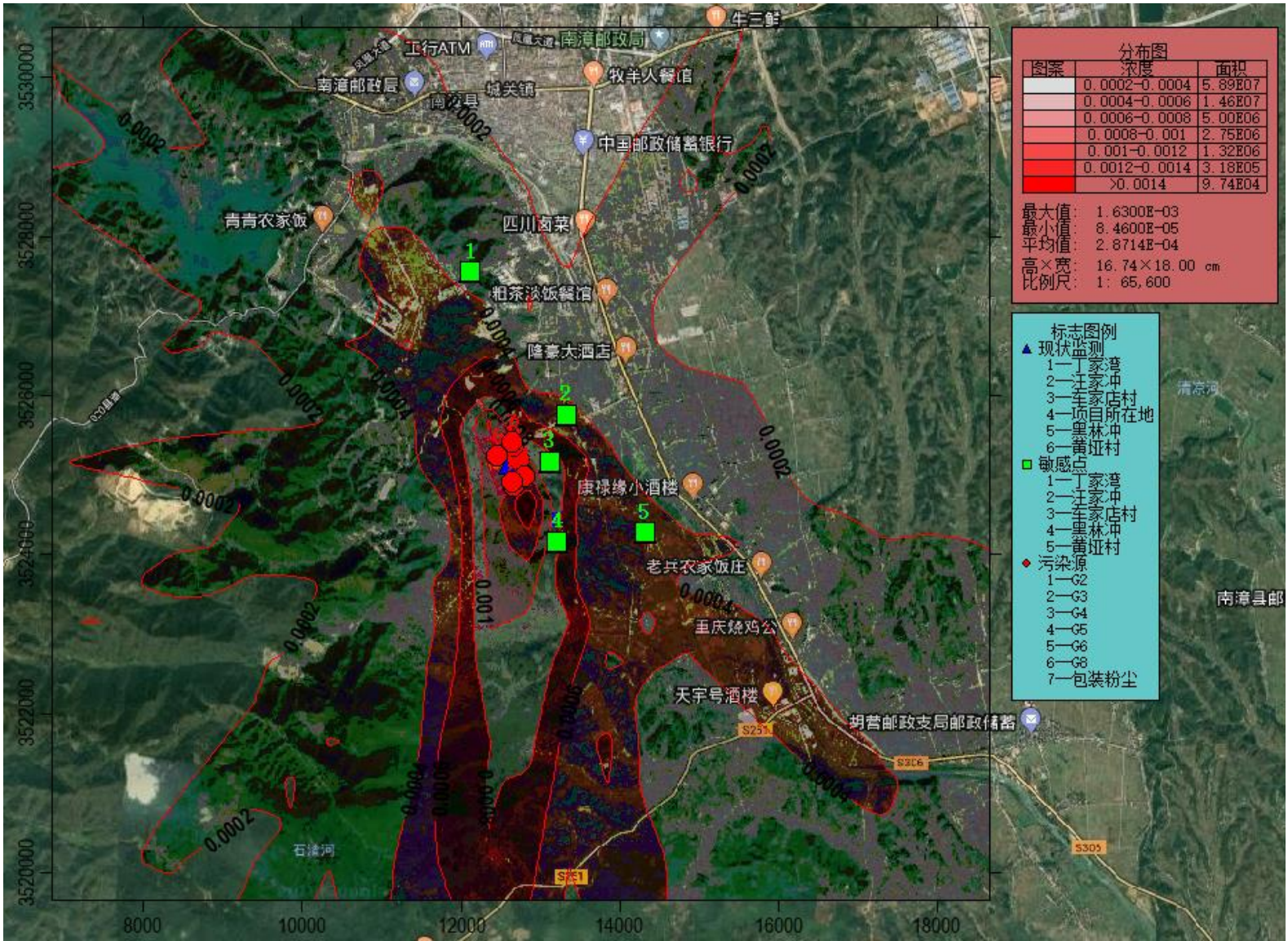
图 5.1-2b 未叠加背景值后 PM2.5 一次污染物最大落地浓度日平均浓度贡献值等浓度线图
