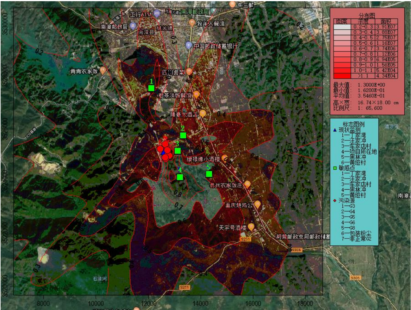
图 5.1-11b 非正常工况叠加背景值 PM_{10} 最大落地浓度小时平均浓度贡献值等浓度线图
