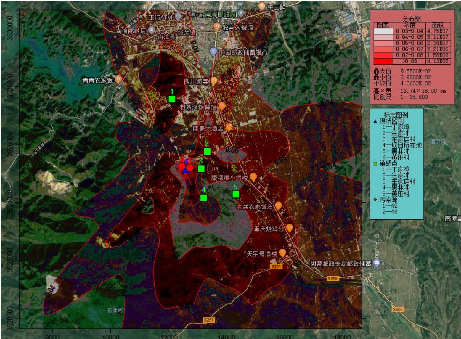
图 5.1-7a 叠加背景值后 NO 2 最大落地浓度小时平均浓度贡献值等浓度线图
