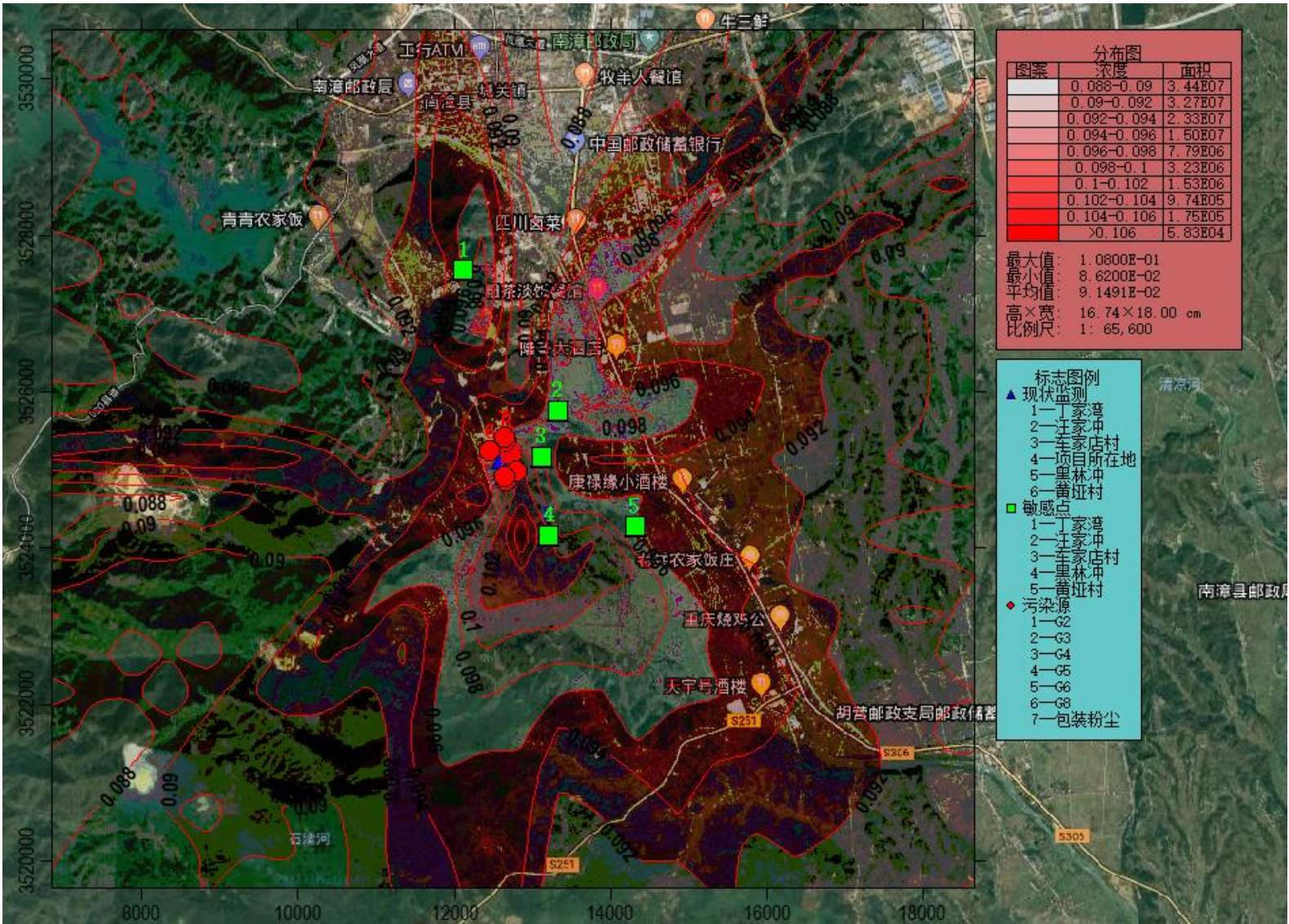
图 5.1-8a 叠加背景值后 PM 10 最大落地浓度小时平均浓度贡献值等浓度线图
