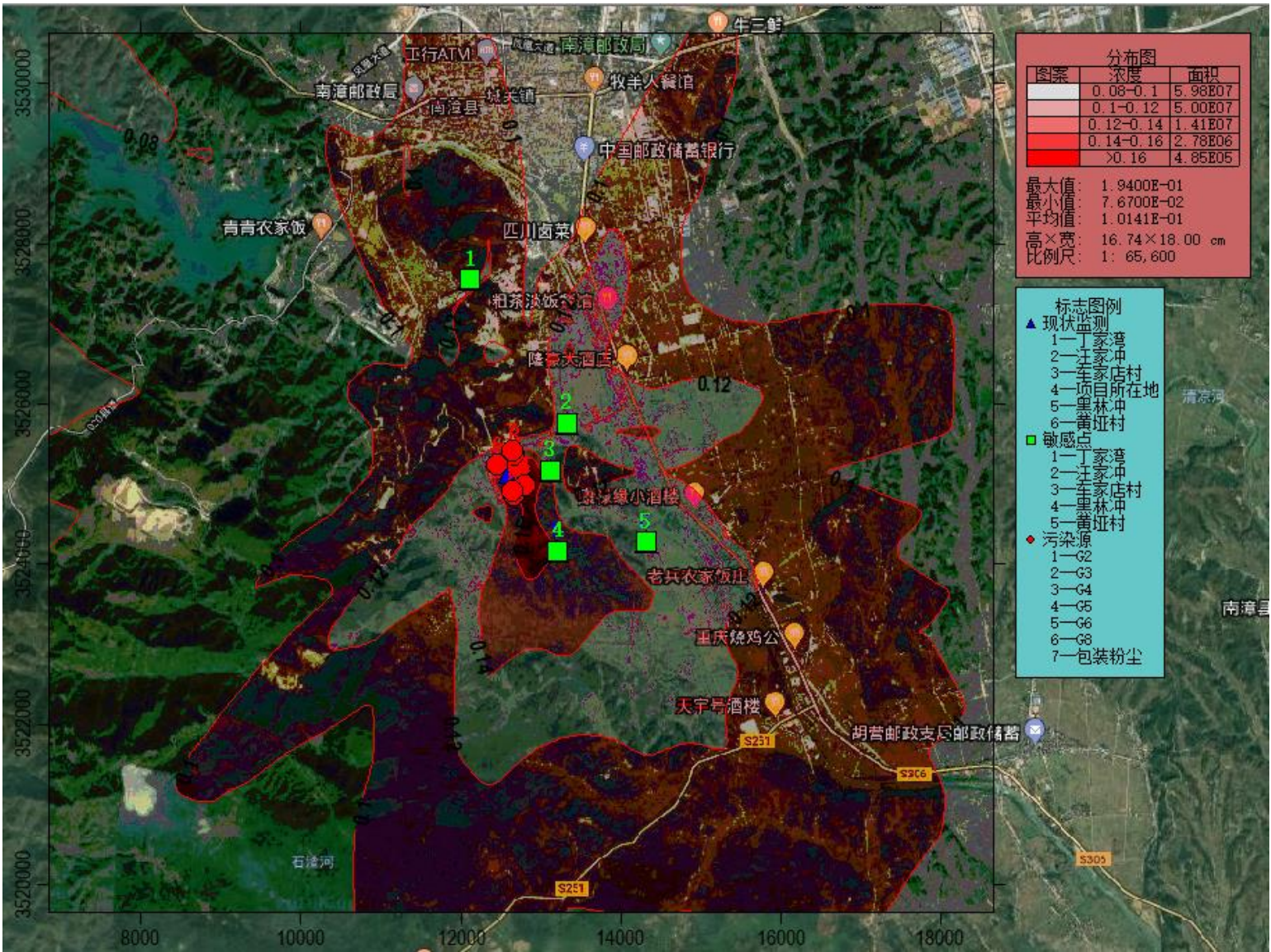
图 5.1-3a 叠加背景值后 PM2.5 二次污染物最大落地浓度年平均浓度贡献值等浓度线图
