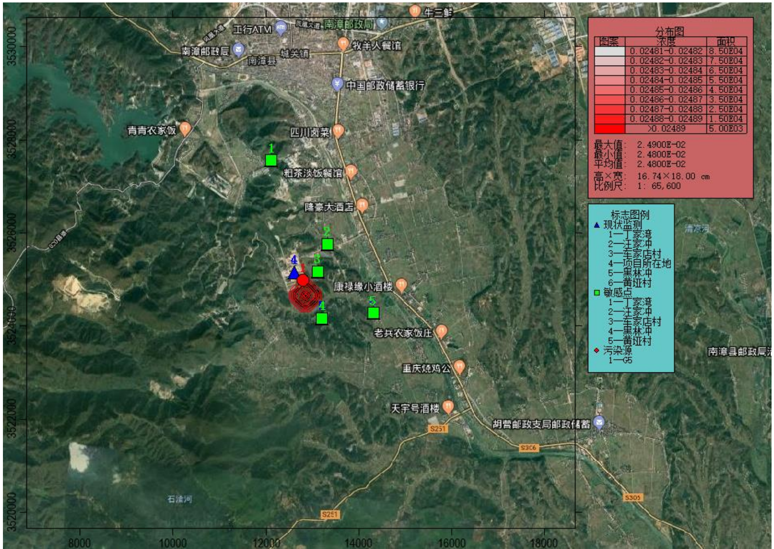
图 5.1-6a 未叠加背景值后 HCl 最大落地浓度日平均浓度贡献值等浓度线图
