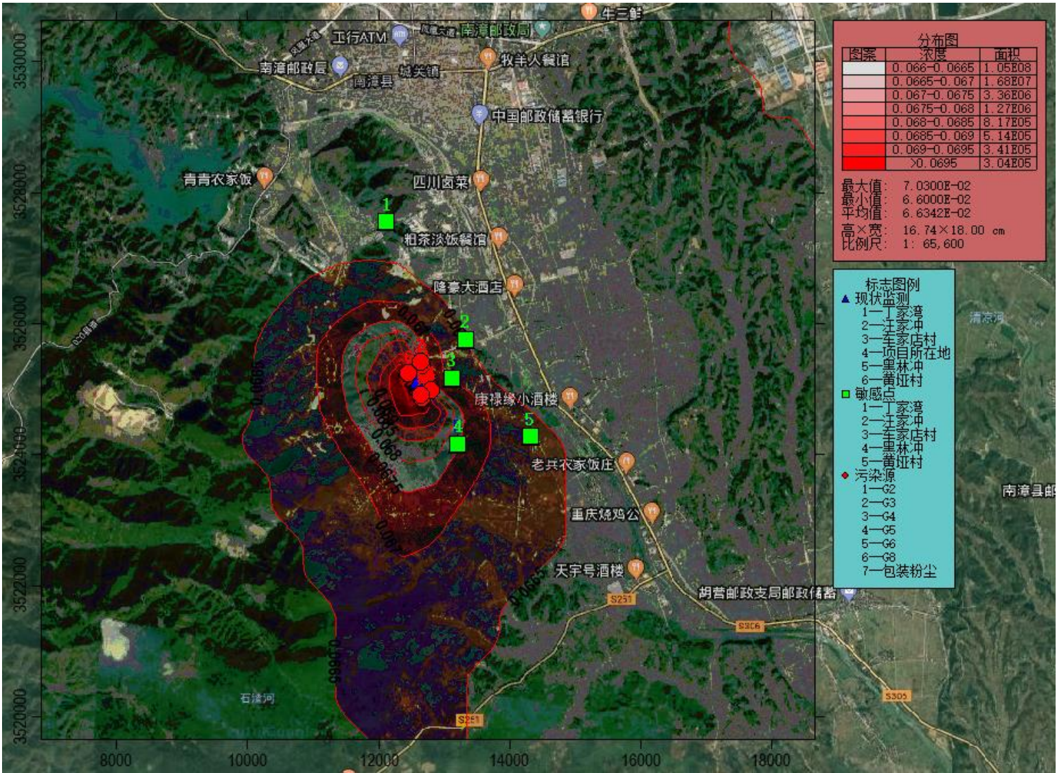
图 5.1-4c 未叠加背景值后 PM2.5 二次污染物最大落地浓度年平均浓度贡献值等浓度线图
