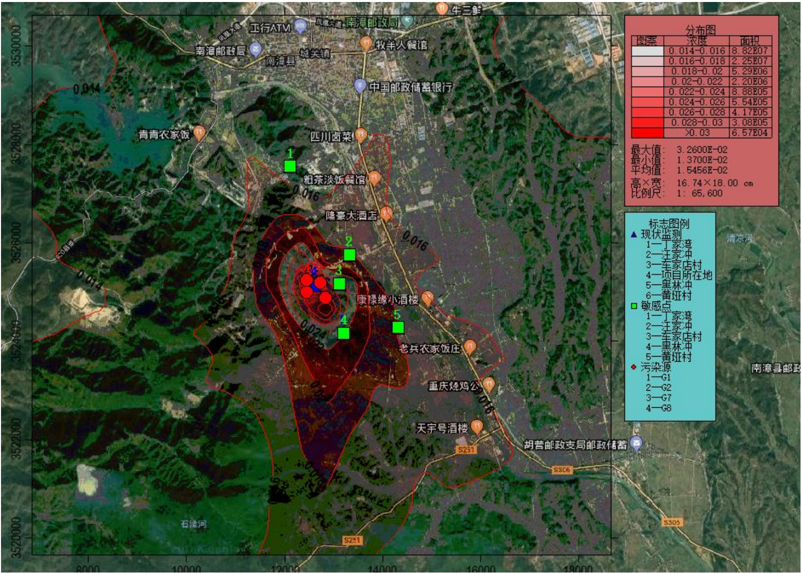
图 5.1-9b 叠加背景值 SO 2 最大落地浓度日平均浓度贡献值等浓度线图
