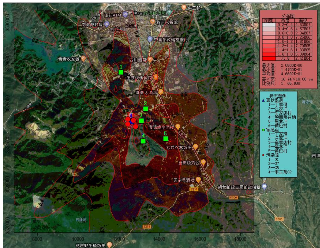
图 5.1-11a 非正常工况叠加背景值 SO 2 最大落地浓度小时平均浓度贡献值等浓度线图
