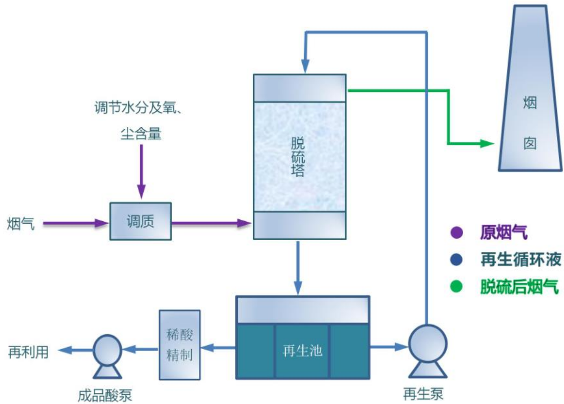
图 6.2-1 硫酸烟气脱硫工艺流程示意图
