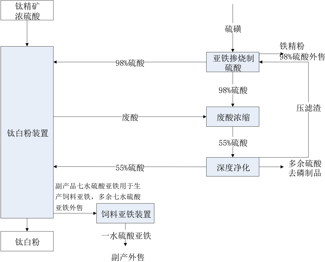
图 2.2-1 产品流向图
