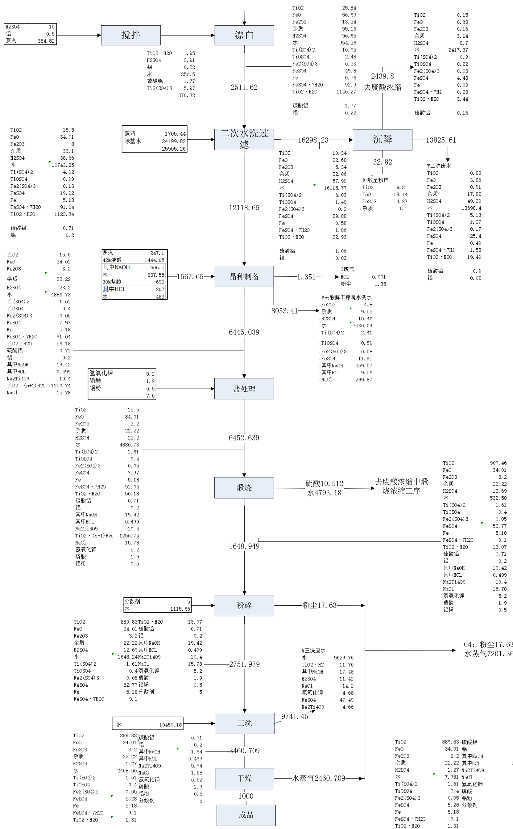
图 2.3-1 钛白粉生产装置总物料平衡图 （单位：kg/t 钛白粉）
