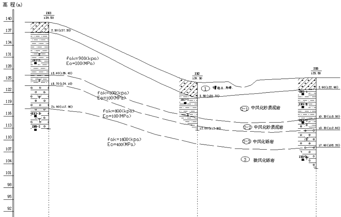
图 5.4-3 工程地质剖面图 2
