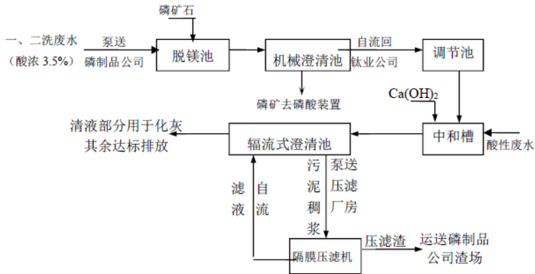
图 6-3 酸性废水处理工艺流程图
