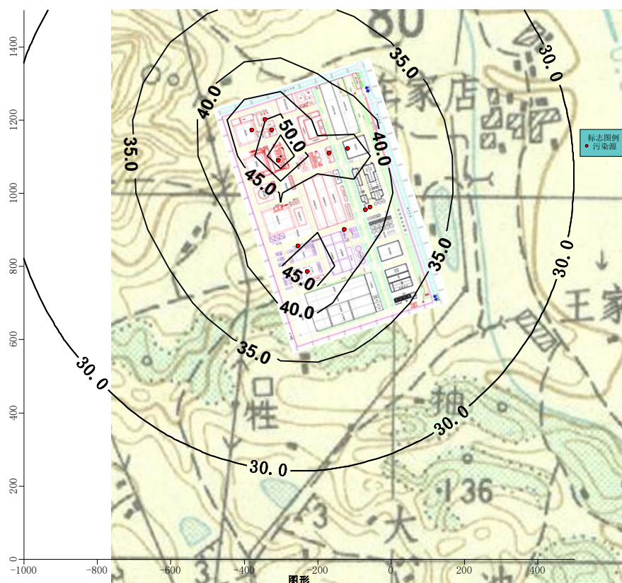
图 5.2-1 噪声贡献值等值线分布图
